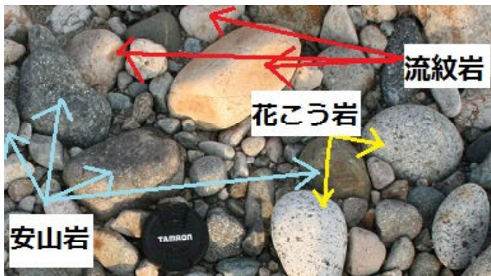
おもな岩石の種類
